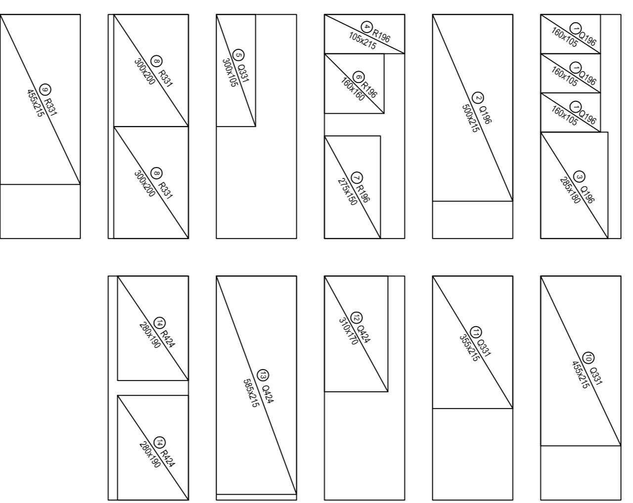
Razrez armaturnih mrež
