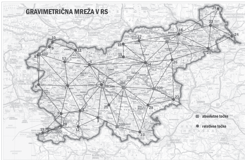
Slika 3: Idejna zasnova nove gravimetrične mreže 1. reda Republike Slovenije.
