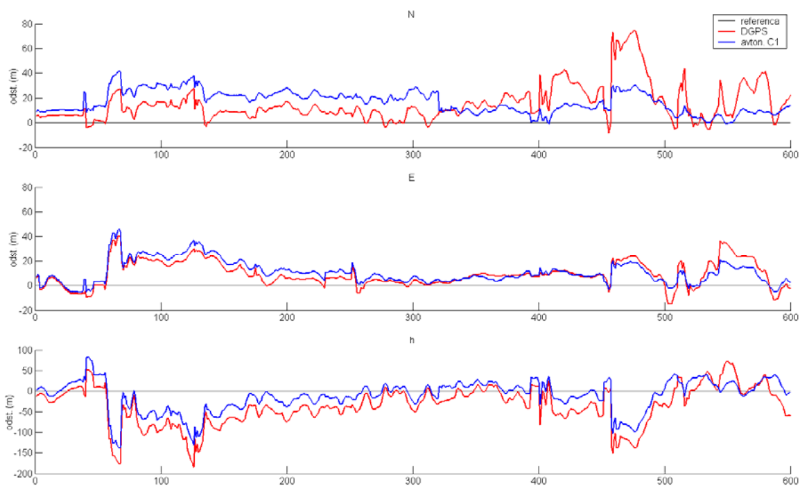
Slika 4-6: DGPS v oteženih pogojih
