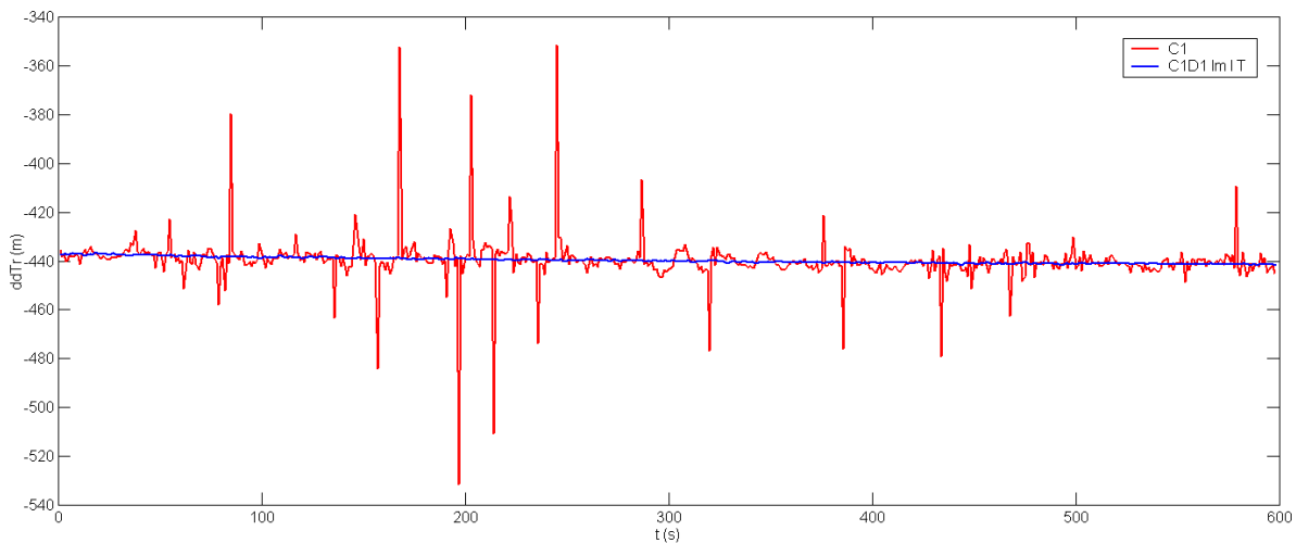
Slika 4-48: Spremembe sprejemnikove ure v najslabši in v najboljši rešitvi znotraj objekta
