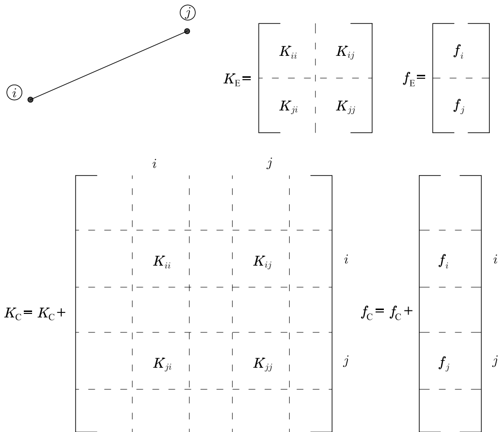
Slika 2.6: Shema sestavljanja tangentne matrike konstrukcije.
