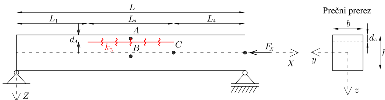
Slika 6.13: Delaminirani nosilec z vzmetmi med lamelama.
