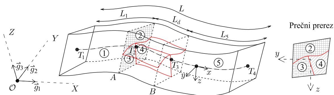
Slika 5.1: Model nosilca z dvema delaminacijama enake dolžine.
