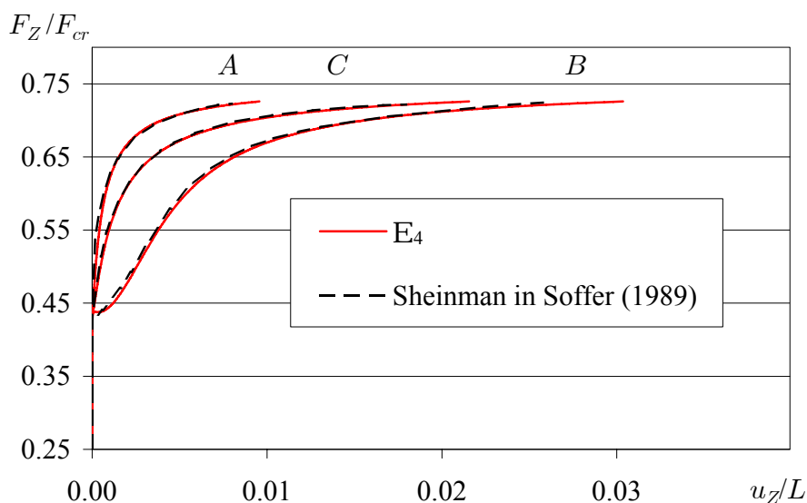
Slika 5.11: Obtežno deformacijska postkritična pot karakterističnih točk na delaminiranem nosilcu. Figure 5.11: Load deflection paths of characteristic points of delaminated beam.
