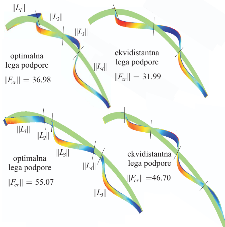
Slika 7.6: Krožni lok s H_{rel} = 0.2 . Uklonske oblike in normirani kritični obtežni faktorji za optimalno in ekvidistantno podprt lok (tri in štiri podpore).
