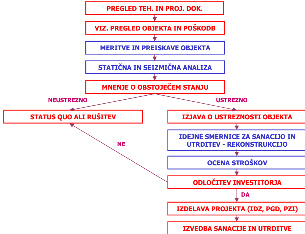
Slika 3.1: Diagram poteka aktivnosti pri utrditvi (zidane) zgradbe
