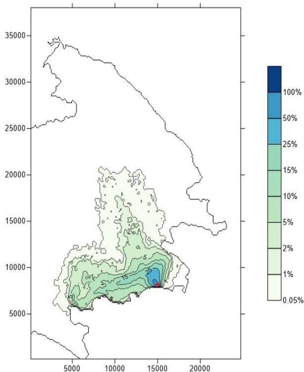
Slika 2: Verjetnosti pojava naftnega madeža pri razlitju v bližini koprskega pristanišča med 19. in 21. 3. 2009, pridobljene po metodi trajektorij. Mesto razlitja je označeno z rdečo.
