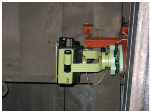
Slika 6: Navezava na reper RJ27 v jami (levo zgoraj), na reper JEK na površini (desno zgoraj), reflektor na nosilcu tik pod odvoziščem na jašku NOP – pogled od zgoraj proti jami (levo spodaj) in instrument na isti merski točki kot prej reflektor – pogled od strani (desno spodaj).
