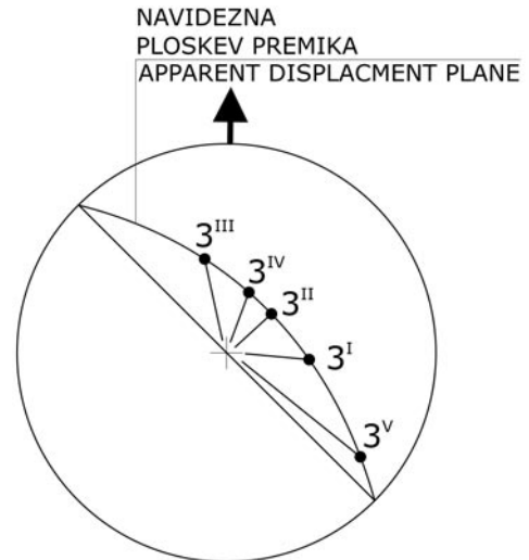
Sl. 5. Grafična konstrukcija navidezne ploskve premika pri nelinearnem premikanju po več izmerah
