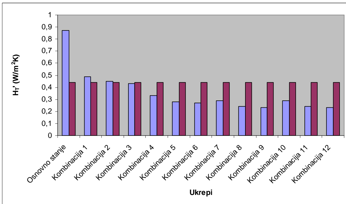
Grafikon 9: Koefficient specifičnih transmissijskih toplotnih izgub stavbe H_T' , kombinacija osnovnih ukrepov
