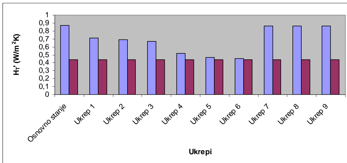
Grafikon 6: Koeficient specifičnih transmisijskih toplotnih izgub stavbe H_T' , osnovni ukrepi
