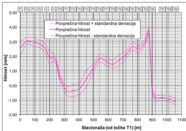
Slika 16: Potek vzdolžnih hitrosti vzdolž desnega brega obtočnega kanala gradbene jame pri Q_{10} = 2560 \text{ m}^3/\text{s} .
