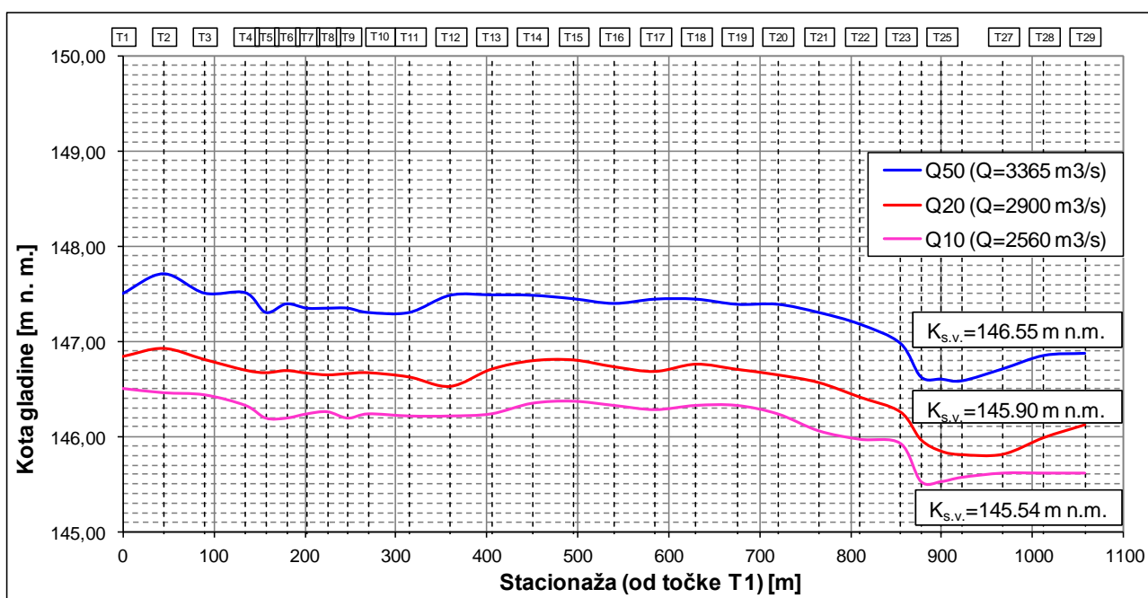
Slika 15: Vz dolžni potek gladin ob desnem bregu obtočnega kanala.
