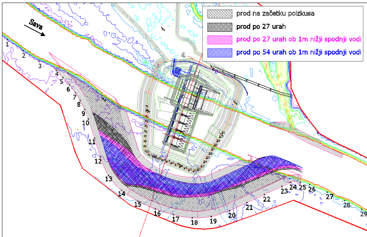
Slika 12: Primerjava erozije v obtočnem kanalu med različnimi poizkusi. Pretok Q = 1800 \text{ m}^3/\text{s} .
