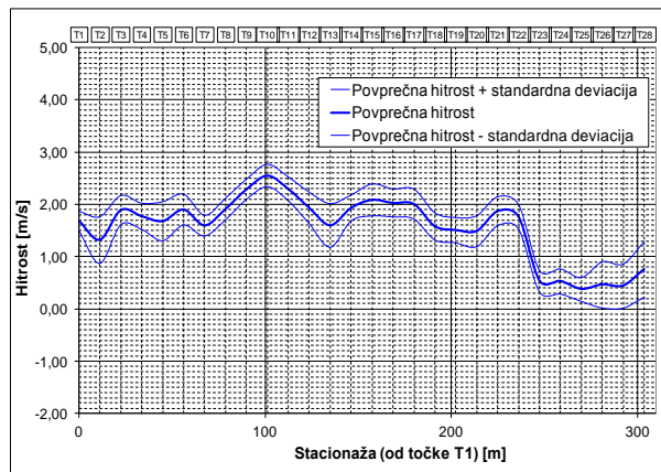
Slika 21: Potek vzdolžnih hitrosti vzdolž nasipa gradbene jame pri Q_{50} = 3365 \text{ m}^3/\text{s} .
