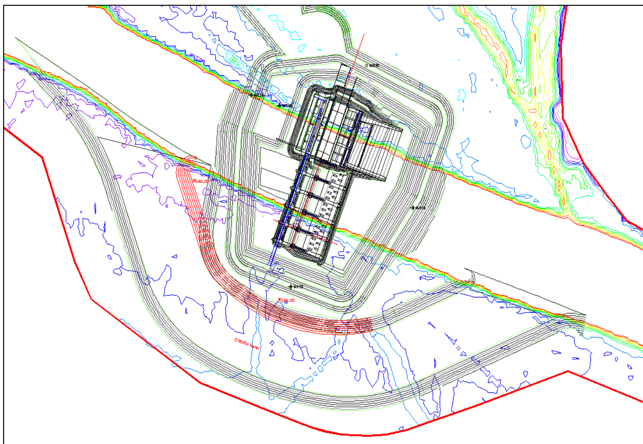
Slika 6: Z rdečimi črtami vrisana predlagana končna oblika obtočnega kanala, ki precej zmanjša potrebne izkope.
