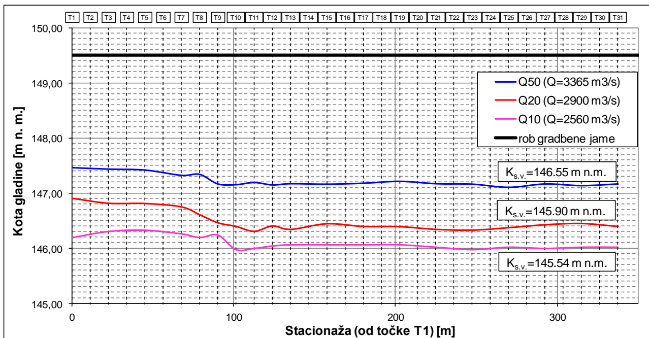
Slika 14: Vz dolžni potek gladin ob gradbeni jami (ob levem bregu obtočnega kanala).
