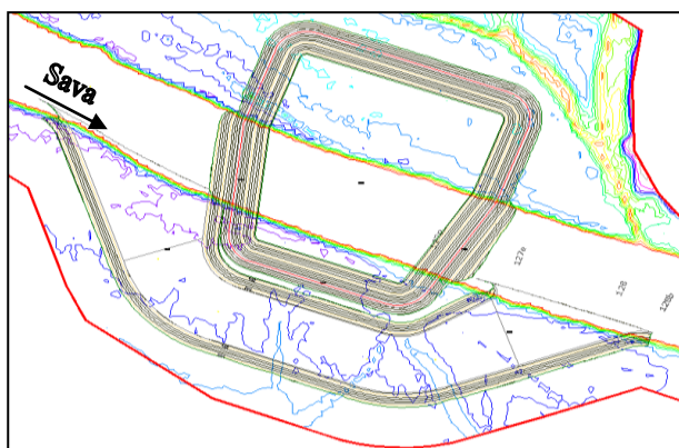
Slika 2: Prva varianta gradbene jame in obtočnega kanala.
