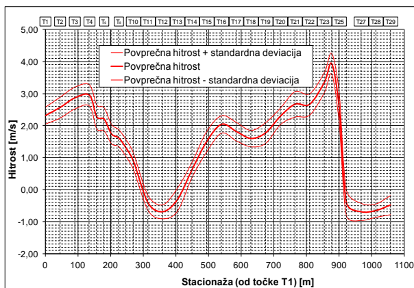
Slika 18: Potek vzdolžnih hitrosti vzdolž desnega brega obtočnega kanala gradbene jame pri Q_{20} = 2900 \text{ m}^3/\text{s} .
