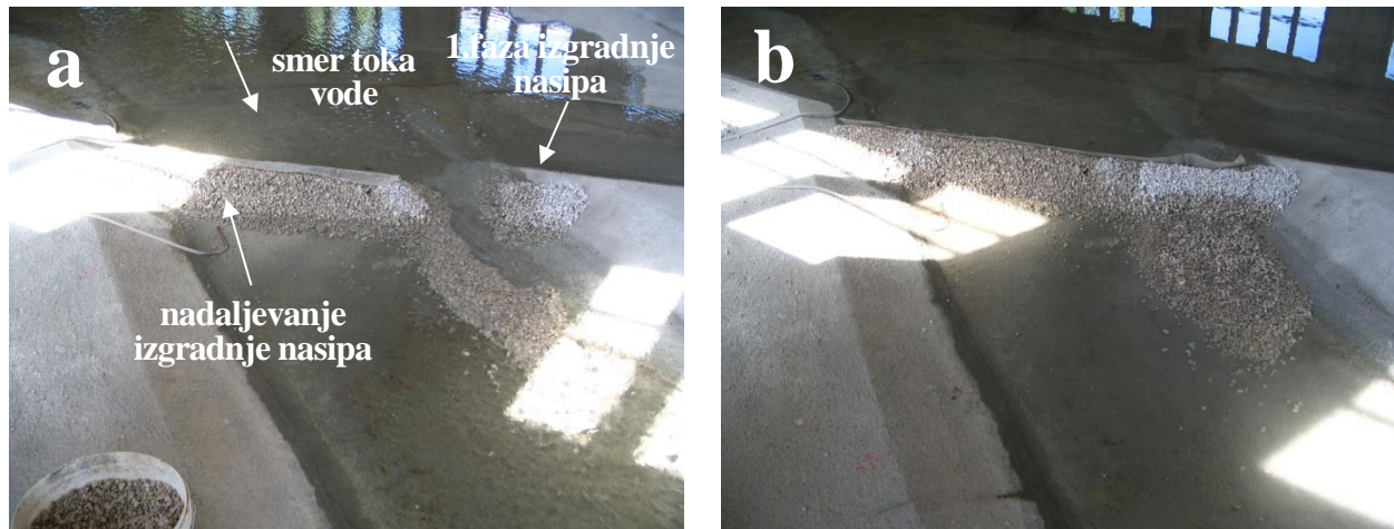
Slika 25: Izgradnja preusmerjevalnega nasipa se prične na levem bregu, zasipanje pa se nadaljuje z desnega brega obtočnega kanala; Q = 200 \text{ m}^3/\text{s} .
