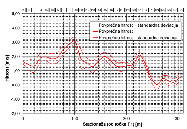
Slika 19: Potek vzdolžnih hitrosti vzdolž nasipa gradbene jame pri Q_{20} = 2900 \text{ m}^3/\text{s} .
