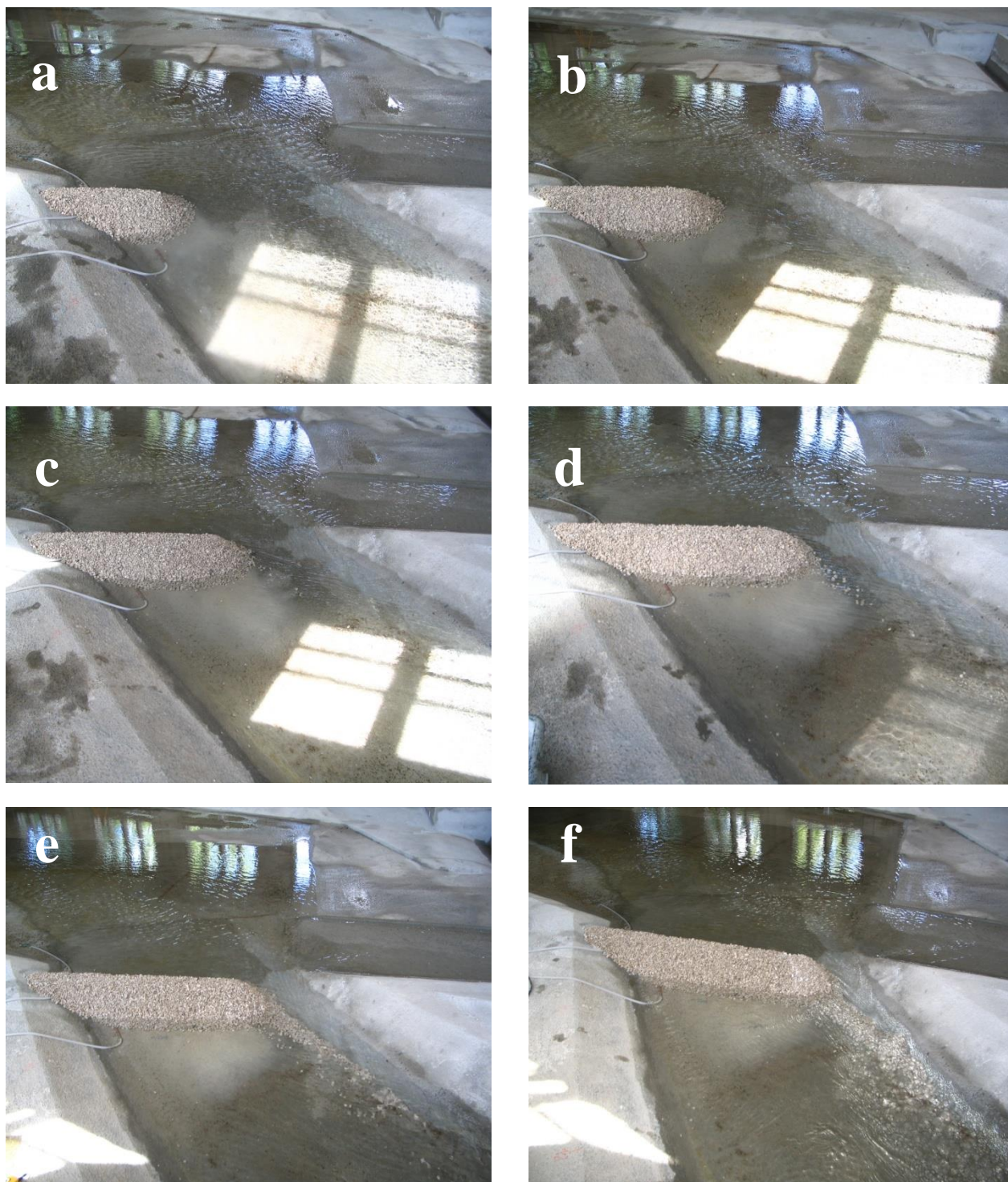
Slika 24: Napredovanje izgradnje preusmerjevalnega nasipa od desnega proti levemu bregu obtočnega kanala v primeru dveh znižanih prelivnih polj pregrade in pretoku Q = 200 \text{ m}^3/\text{s} .
