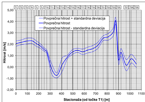
Slika 20: Potek vzdolžnih hitrosti vzdolž desnega brega obtočnega kanala gradbene jame pri Q_{50} = 3365 \text{ m}^3/\text{s} .
