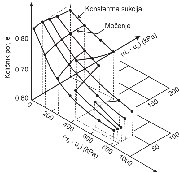
Slika 8.7: Količnik por v odvisnosti od sukcije in sferične napetosti v izotropnem stanju (Matyas in Radhakrishna, 1968, citat po Fredlund in Rahardjo, 1993).
