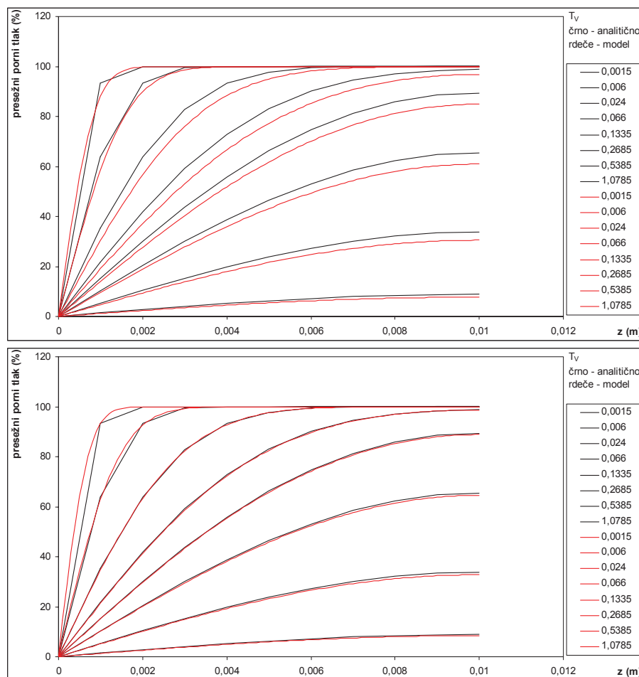
Slika 14.26: Presežni porni tlaki med bremensko stopnjo za primer izračuna s korakom od 1 do 60 s (zgoraj) ter za korak 1 s (spodaj).
