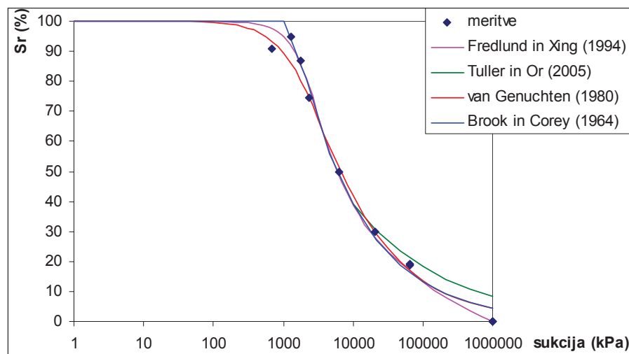
Slika 14.7: Opis meritve z različnimi funkcijami za opis retencijske krivulje.
