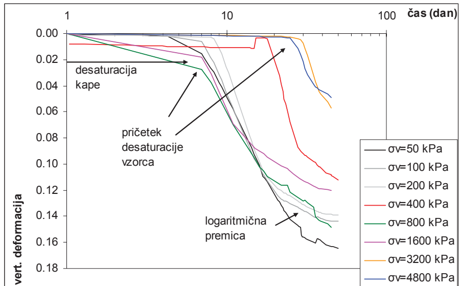
Slika 13.7: Časovni razvoj vertikalnih deformacij med sušenjem v edometru. Figure 13.7: Development of vertical deformations vs. time in oedometer.
