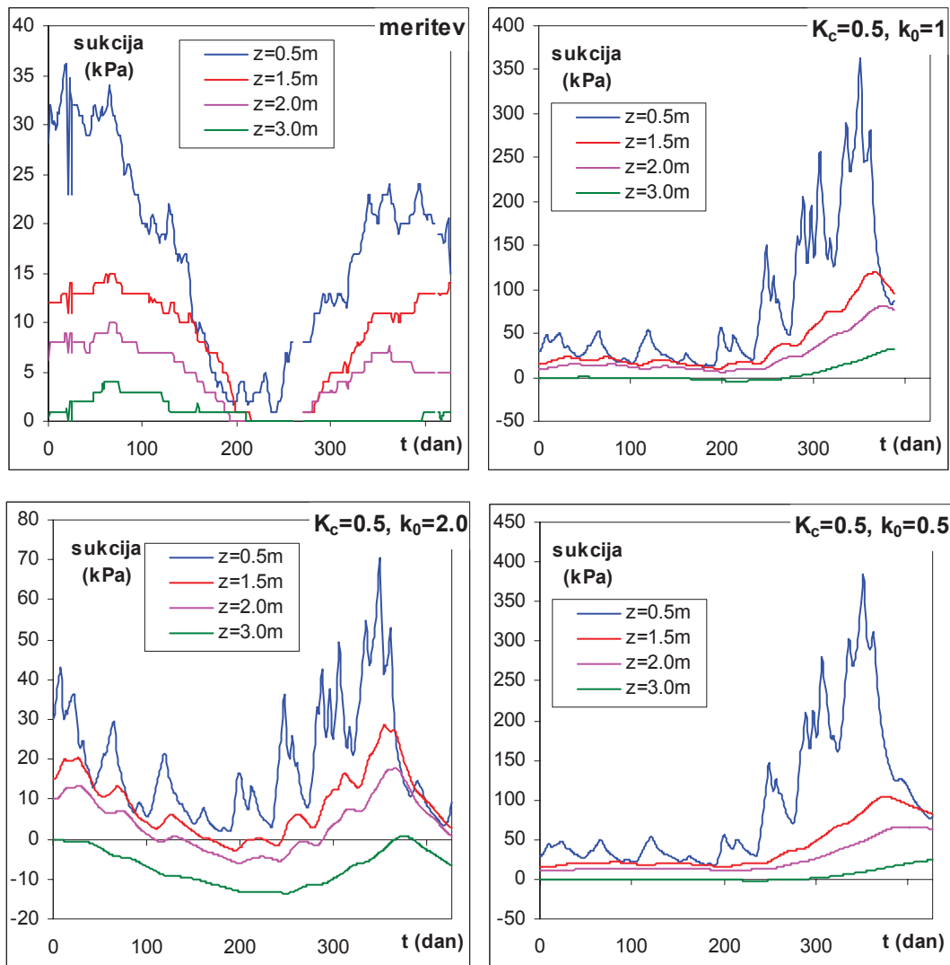
Slika 14.32: Vpliv vodoprepustnosti v numeričnem modelu na sukcijo v plazini.
