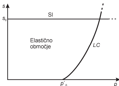
Slika 8.10: Meja tečenja z mejama LC – obremenitev-kolaps in SI – povečanje sukcije (Alonso et al., 1990).
