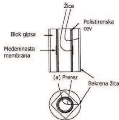
Slika 9.10: Gips blok merilec sukcije (Bulut in Leong, 2008). Figure 9.10: Gips block suction sensor (Bulut and Leong, 2008).
