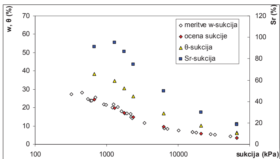
Slika 14.6: Meritve sukcije, vlage in stopnje zasičenosti za primer neobremenjenega vzorca.
