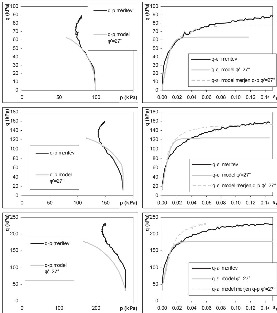
Slika 14.3: CIU meritve v triosni celici in modelna napoved. Po vrsti od zgoraj navzdol si sledijo vzorci: 2002 0.08 mm w = w_L stopnje 100, 200 in 300 kPa.
