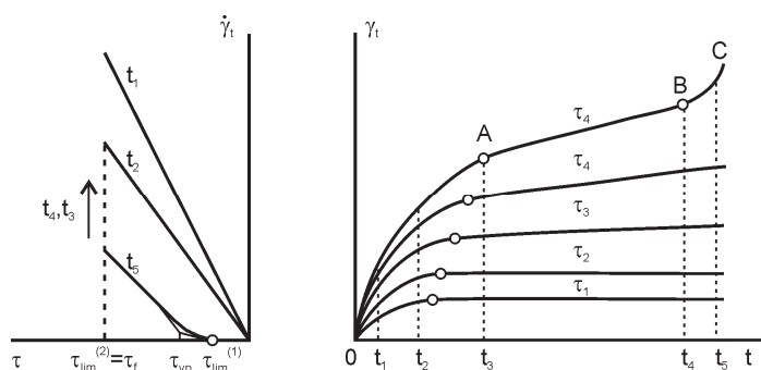
Slika 11.14: Obnašanje glin med preiskavo lezenja v enostavnem strigu (Meschyan, 1995).
