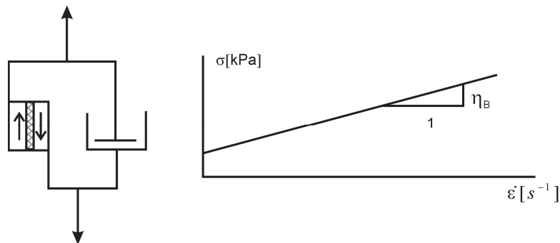
Slika 11.9: Binghamov reološki model in odvisnost napetosti od hitrosti deformacij.
