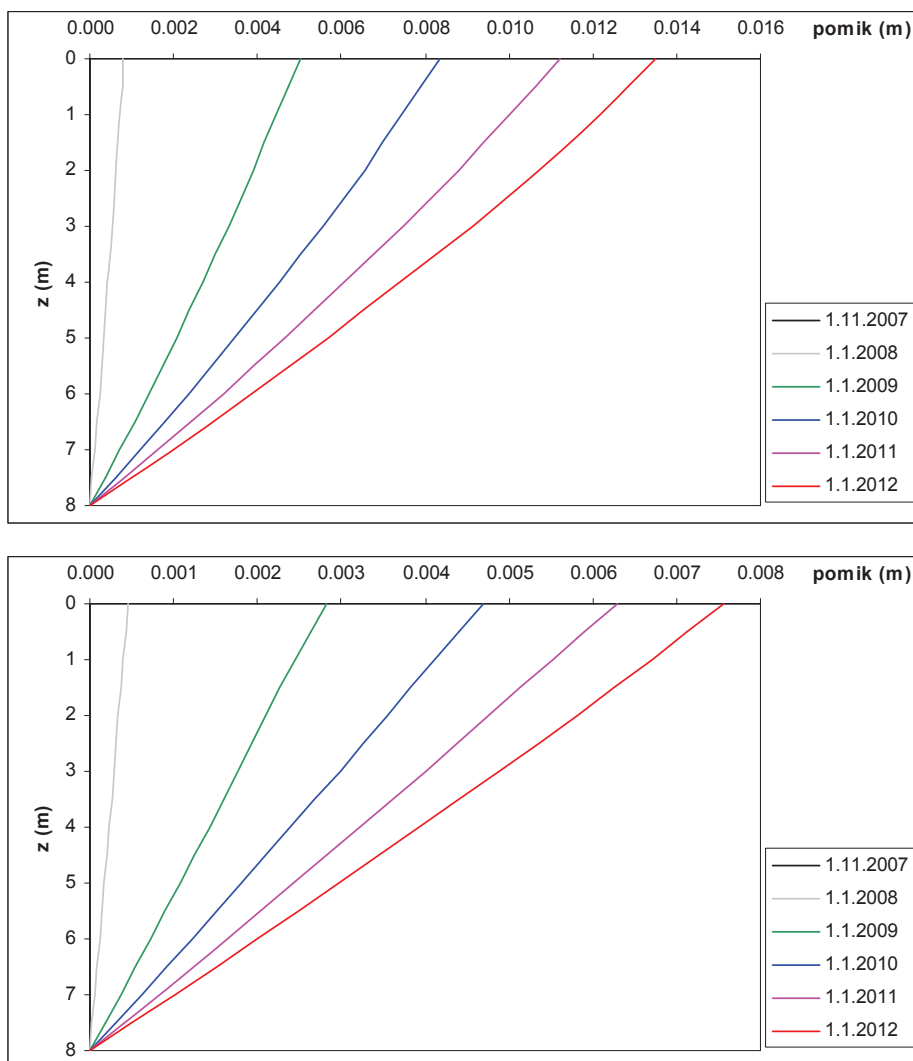
Slika 14.38: Razvoj pomikov v plazini s časom za obdobje 1.11.2007-1.1.2012 za primer z upoštevanjem ugodnih vplivov sukcije. Zgoraj zgornja meja lezenja, spodaj spodnja meja lezenja.
