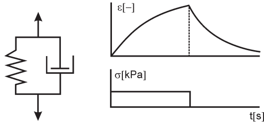
Slika 11.8: Kelvin in Voightov reološki model in odziv na enotsko obremenitev.
