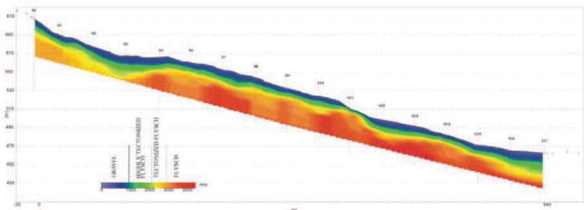
Slika 12.8: Hitrost potresnih valov na vzdolžnem profilu plazu Slano blato (Logar et al., 2005).
