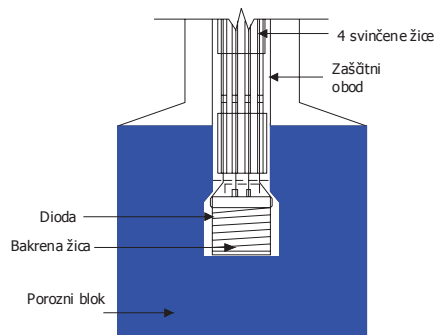
Slika 9.11: Skica merilnika sukcije s toplotno prevodnostjo, dioda služi kot termometer, bakrena žica pa kot grelno telo (Bulut in Leong, 2008).
