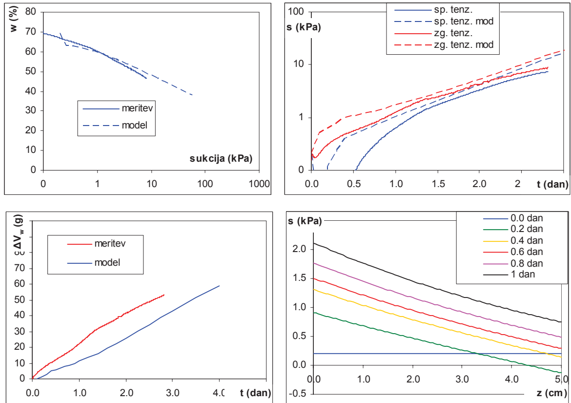
Slika 14.29: Primerjava med meritvijo in rezultati numeričnega modela za primer vzorca HYPROPI.
