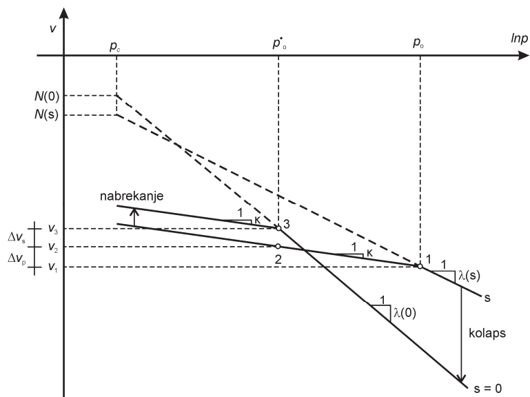
Slika 8.9: Stisljivost zemljine v odvisnosti od sukcije (Alonso et al. 1990).
