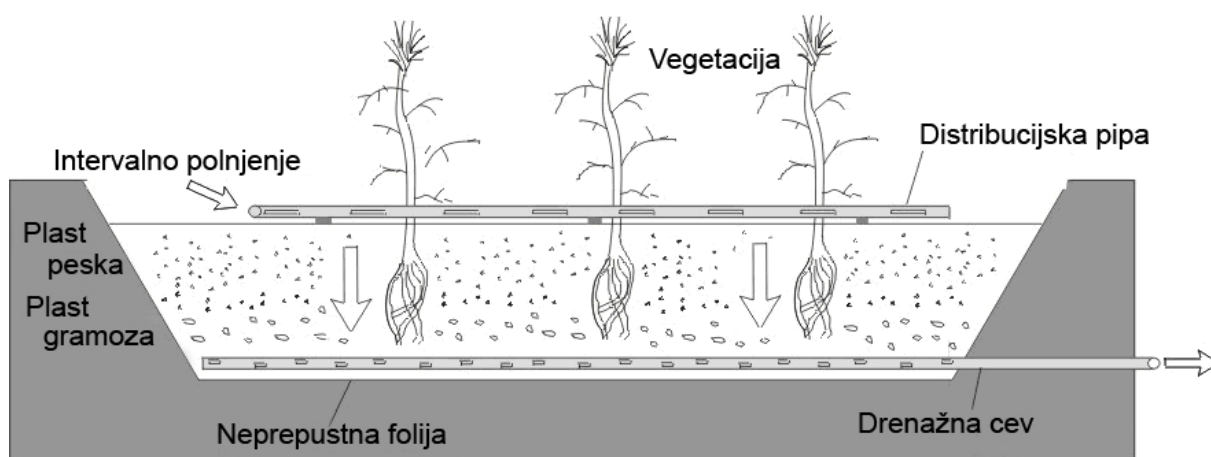
Slika 6: RČN z vertikalnim podpovršinskim tokom vode (Langergraber in Haberl, 2004, cit. po Langergraber, 2008)
