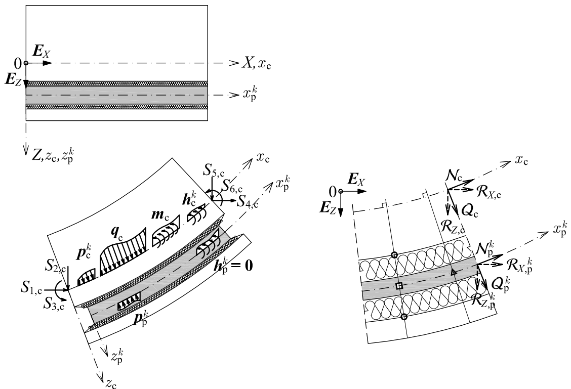
Slika 2.2: Obtežba prednapetega betonskega nosilca.
