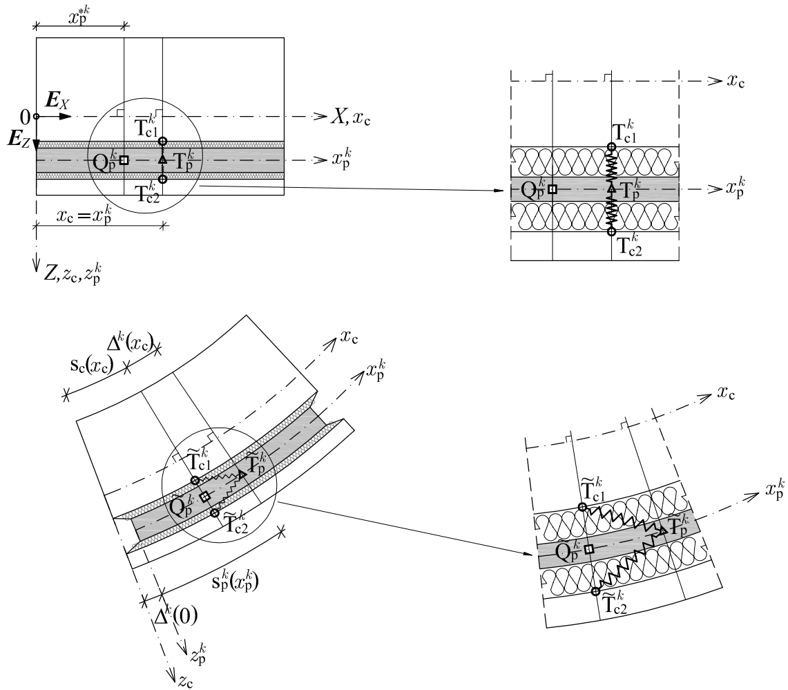
Slika 2.3: Geometrijski pomen zamika na stiku med betonom in prednapetim kablom.
