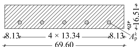
Slika 3.34: Prednapeta betonska plošča s previsi. Geometrijski in materialni podatki ter podatki o obtežbi.
