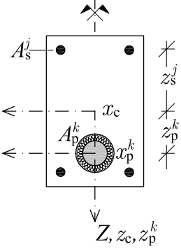
Prečni prerez:
